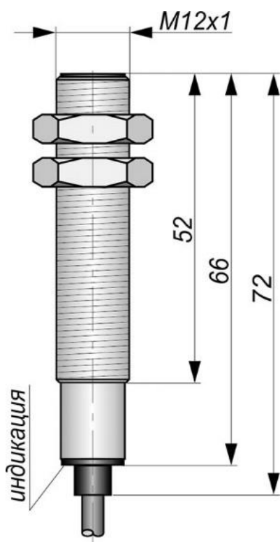
Габаритный чертеж
