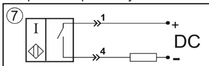
Нормально-разомкнутый контакт
