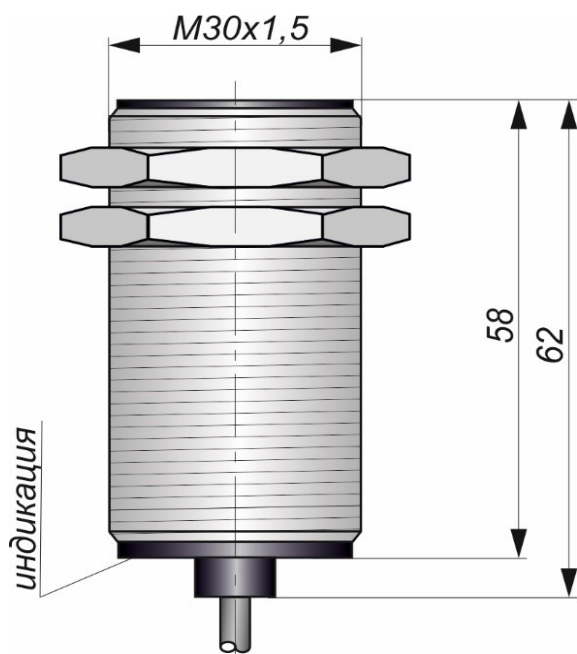
Габаритный чертеж
