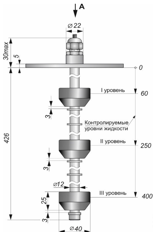
Габаритный чертеж
