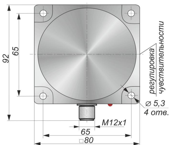
Габаритный чертеж
