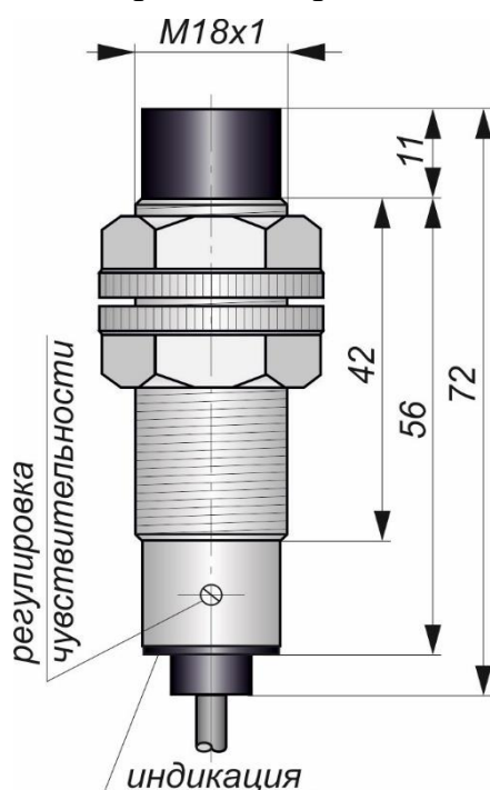
Габаритный чертеж
