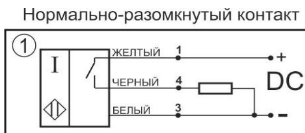
Схема соединения
