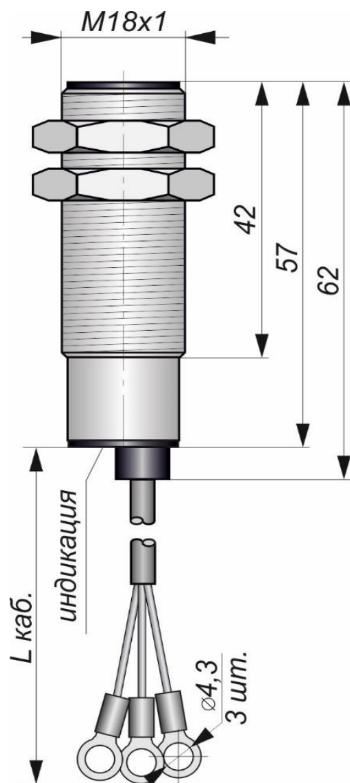
Габаритный чертеж
