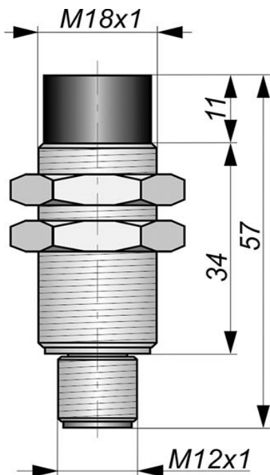
Габаритный чертеж
