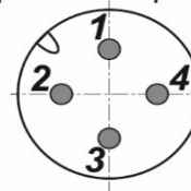
Цоколевка разъема
