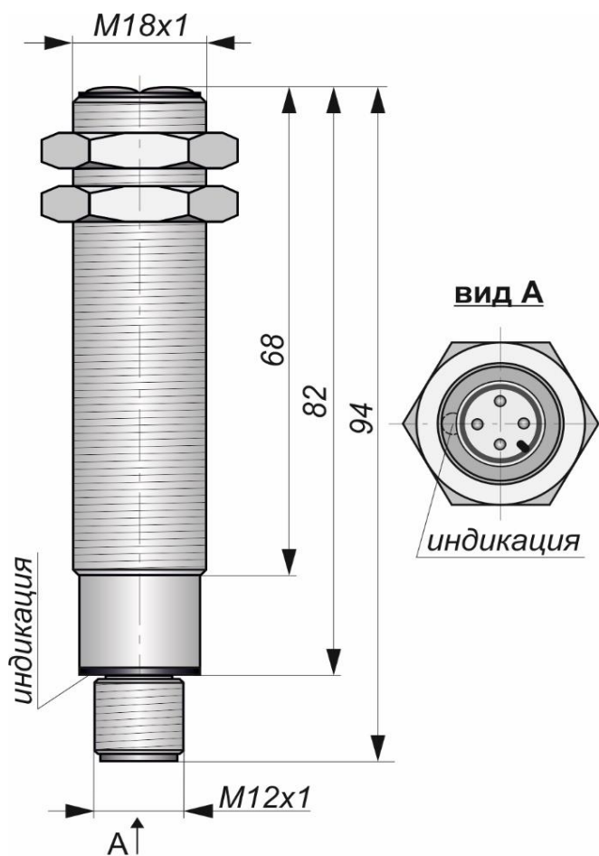
Габаритный чертеж
