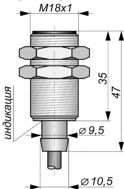
Габаритный чертеж
