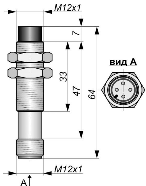
Габаритный чертеж
