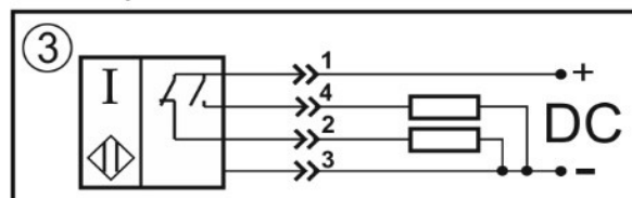
Переключающий контакт
