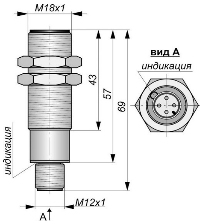
Габаритный чертеж
