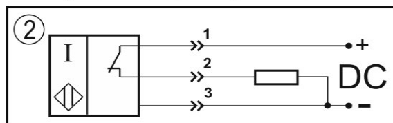
Нормально-замкнутый контакт
