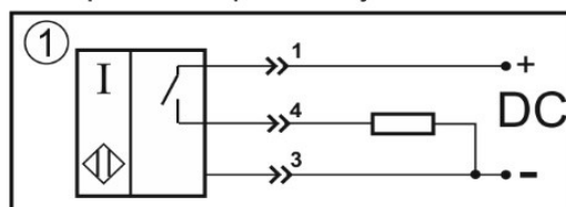
Цоколевка разъема
