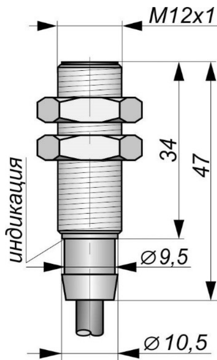
Габаритный чертеж
