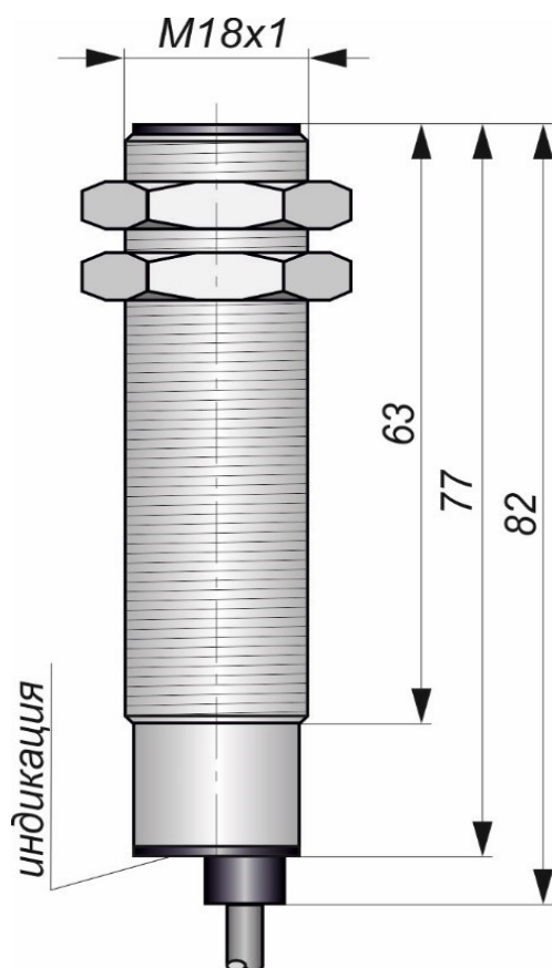
Габаритный чертеж
