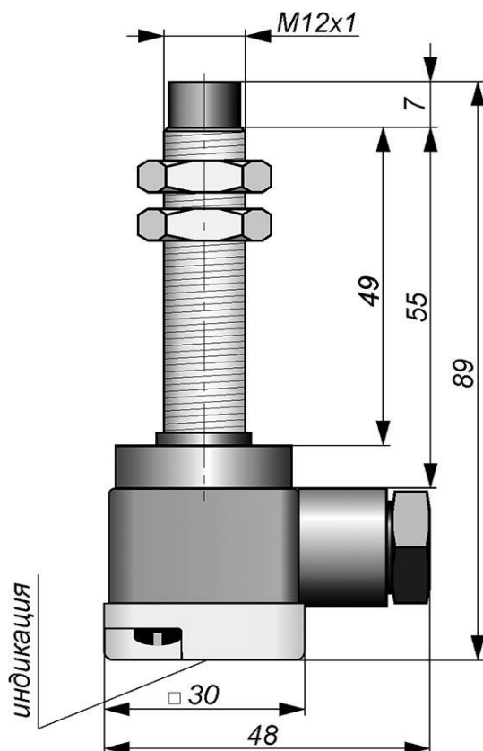
Габаритный чертеж
