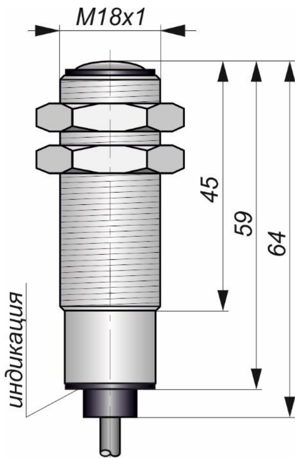
Габаритный чертеж
