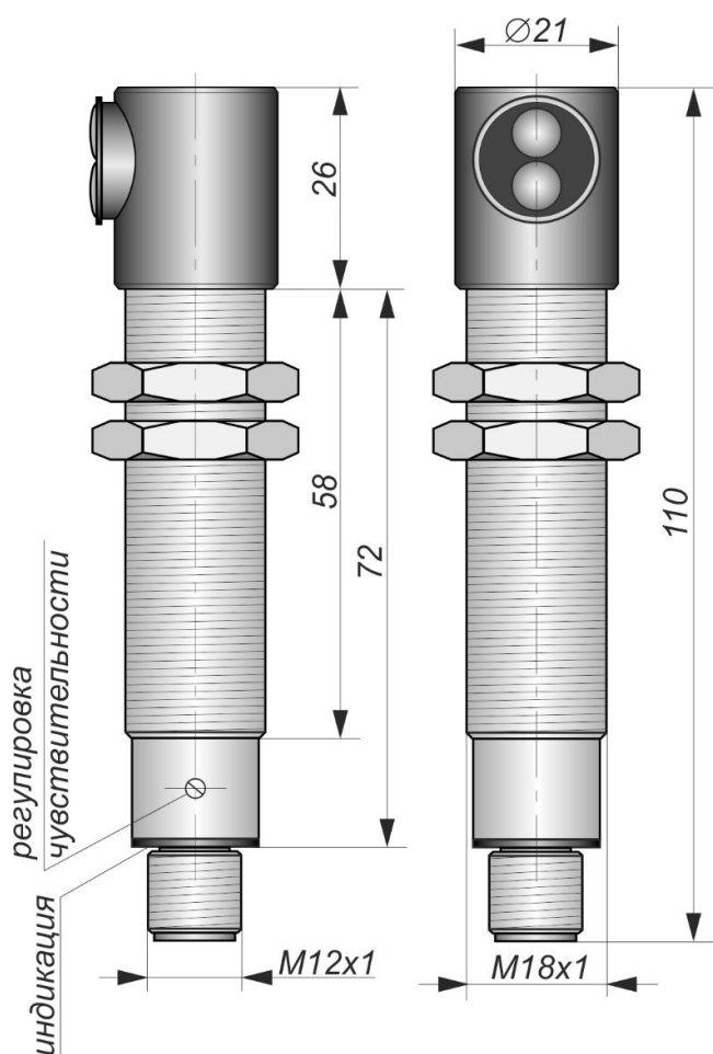
Габаритный чертеж
