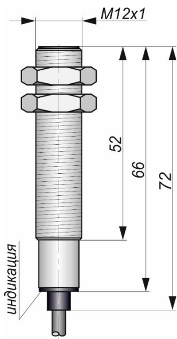
Габаритный чертеж
