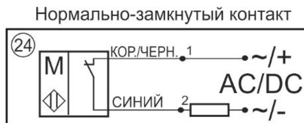
Схема соединения
