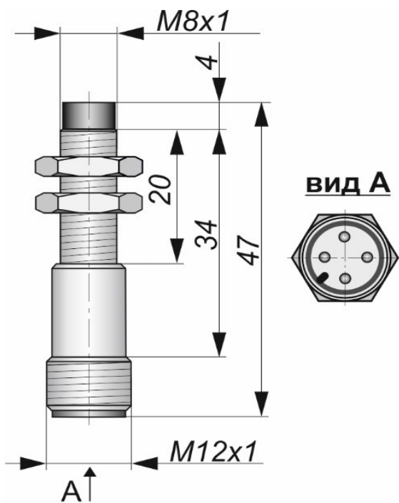
Габаритный чертеж
