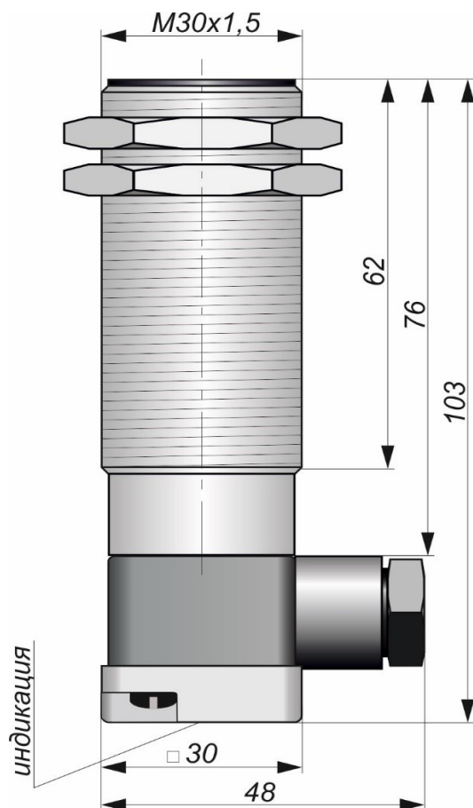
Габаритный чертеж
