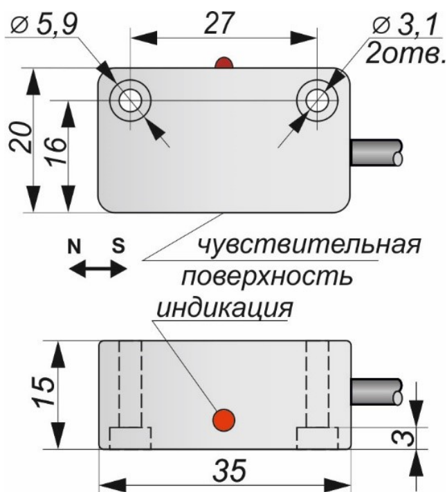
Габаритный чертеж
