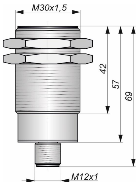
Габаритный чертеж
