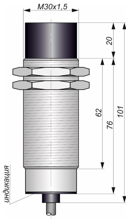
Габаритный чертеж
