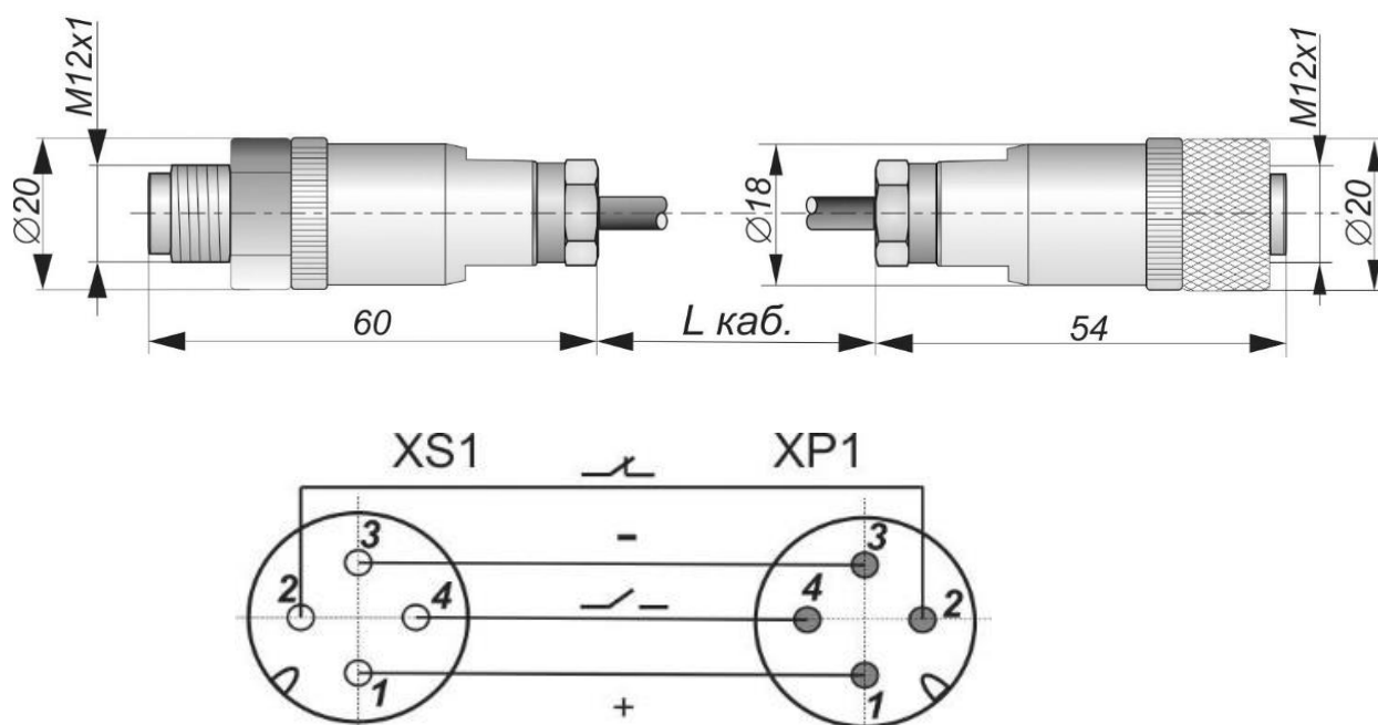
Габаритный чертеж
