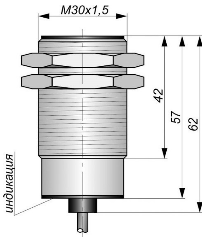
Габаритный чертеж
