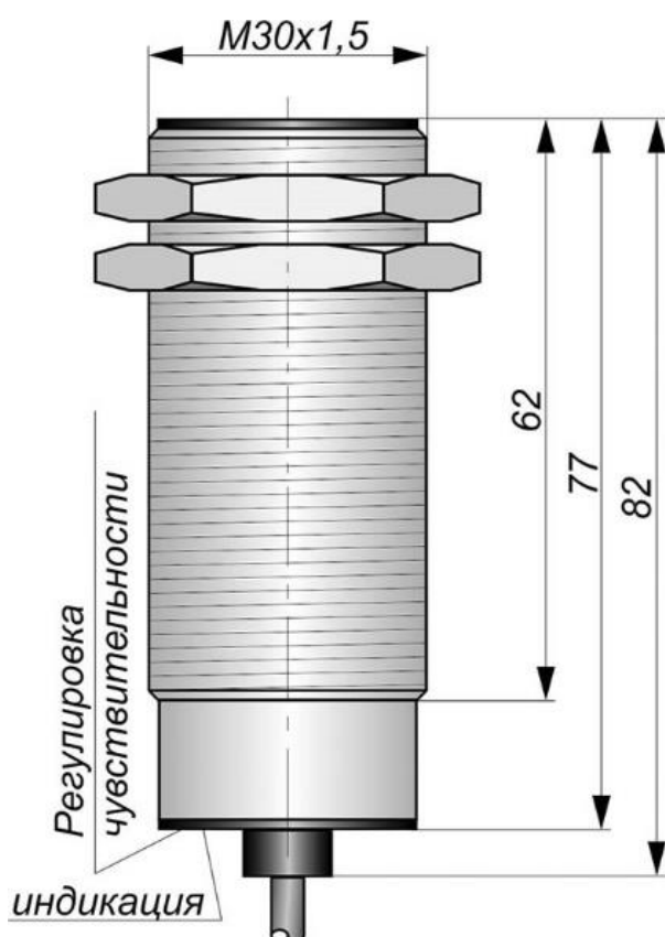
Габаритный чертеж
