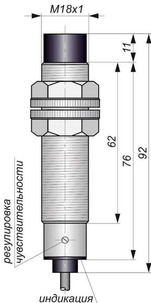
Габаритный чертеж
