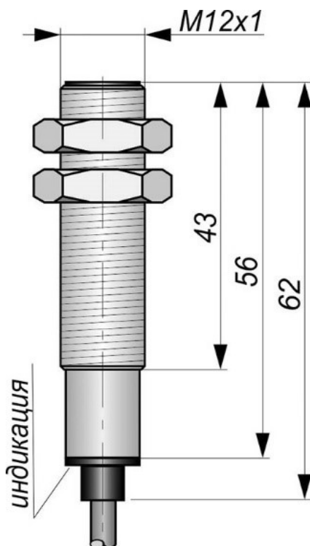
Габаритный чертеж
