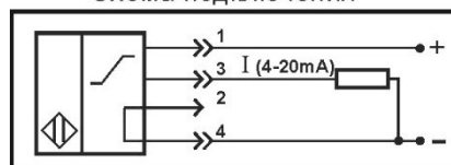
Цоколевка разъема
