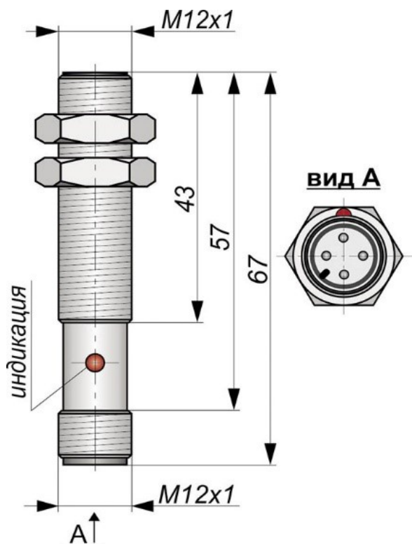
Габаритный чертеж
