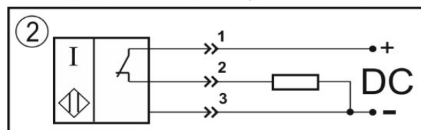
Нормально-замкнутый контакт
