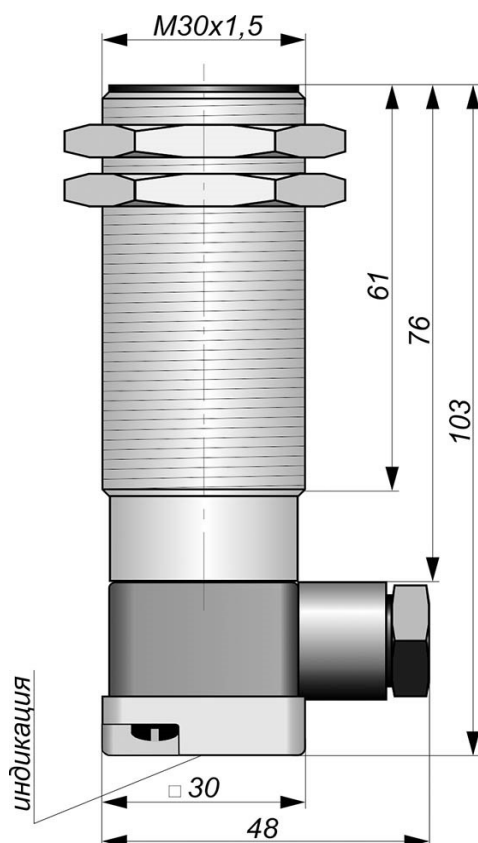
Габаритный чертеж
