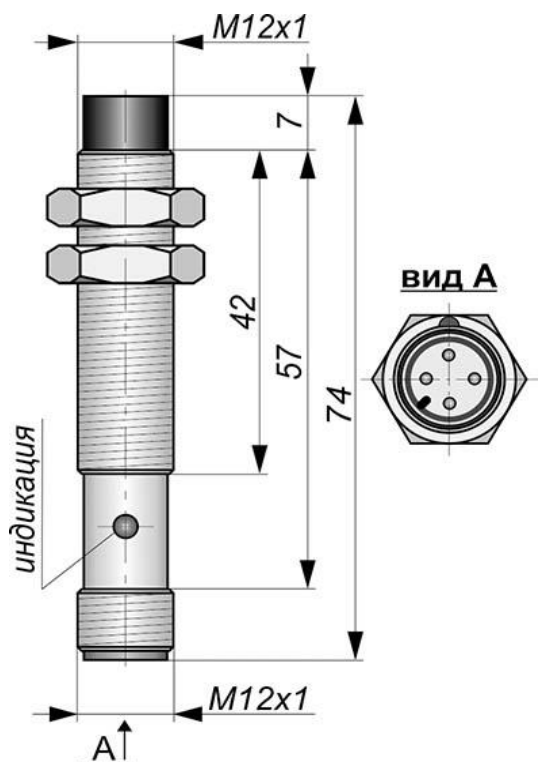
Габаритный чертеж
