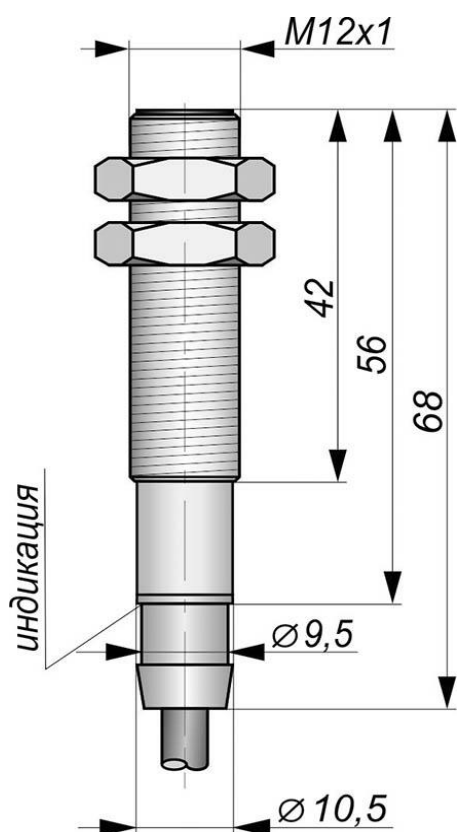
Габаритный чертеж
