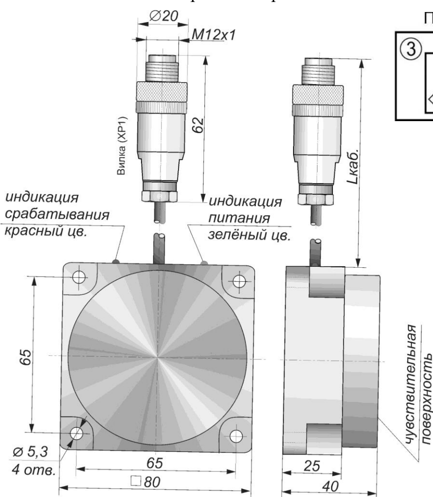
Габаритный чертеж
