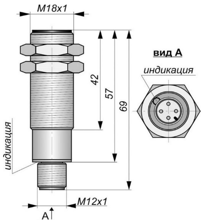
Габаритный чертеж
