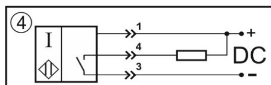
Цоколевка разъема
