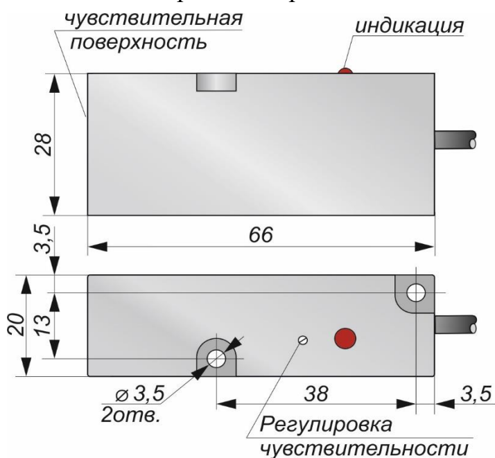
Габаритный чертеж
