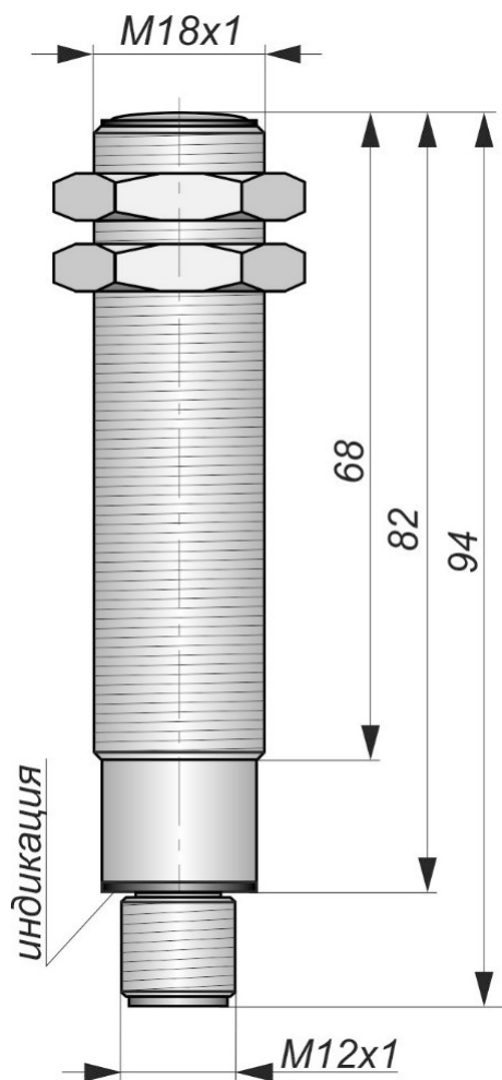
Габаритный чертеж
