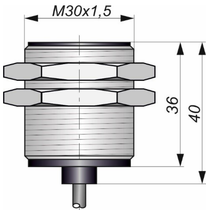
Габаритный чертеж
