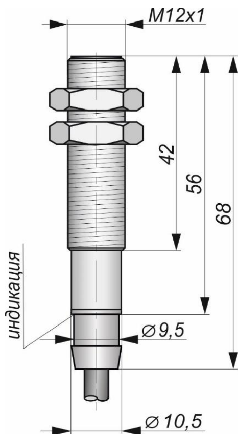
Габаритный чертеж
