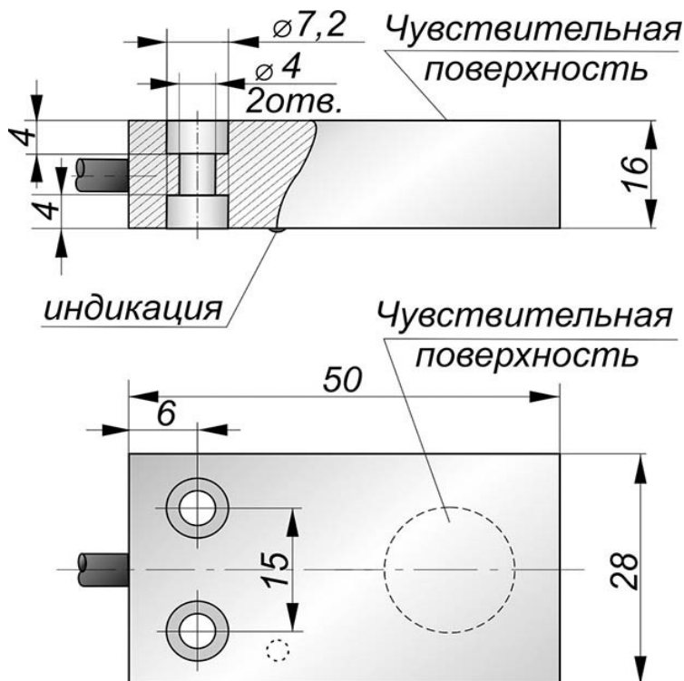
Габаритный чертеж
