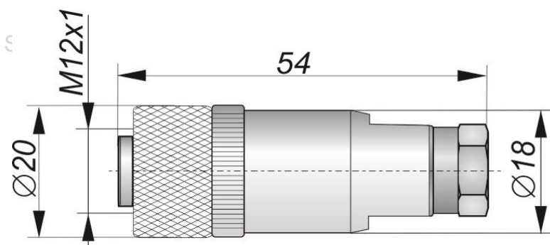
Габаритный чертеж
