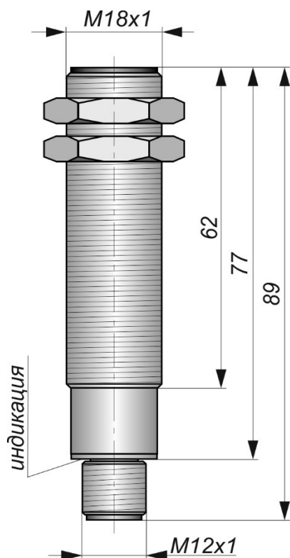
Габаритный чертеж
