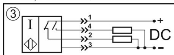
Переключающий контакт
