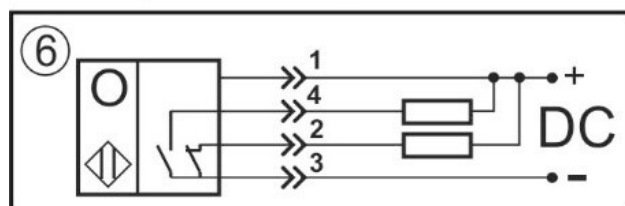
Схема соединения Переключающий контакт
