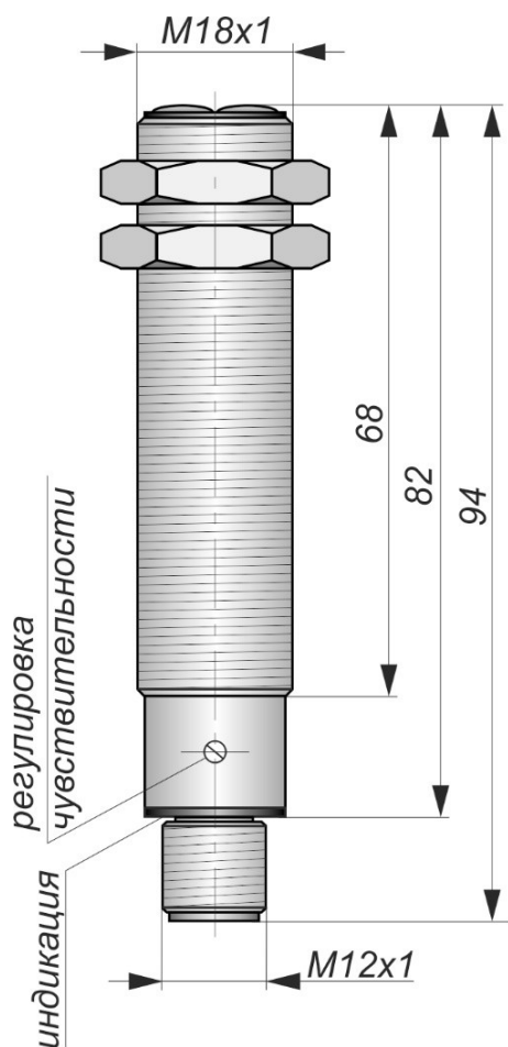
Габаритный чертеж
