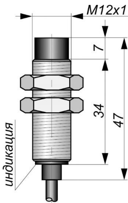
Габаритный чертеж
