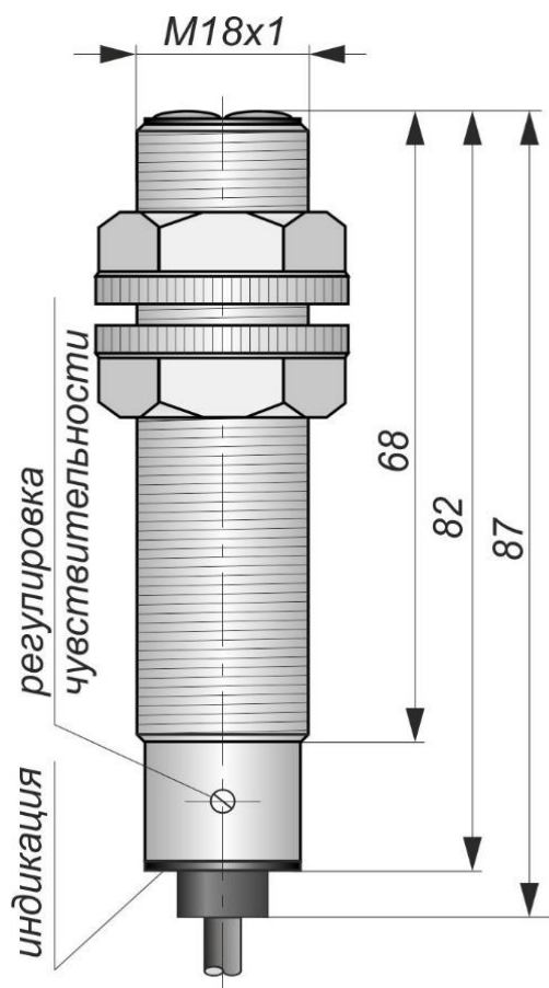
Габаритный чертеж
