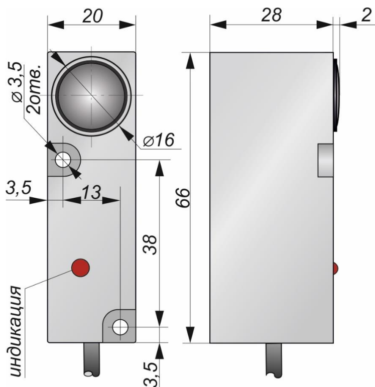
Габаритный чертеж
