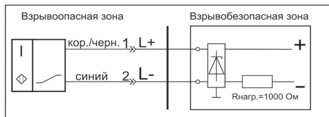
Схема соединения
