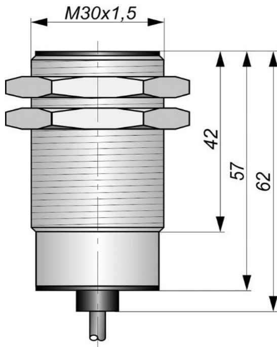
Габаритный чертеж
